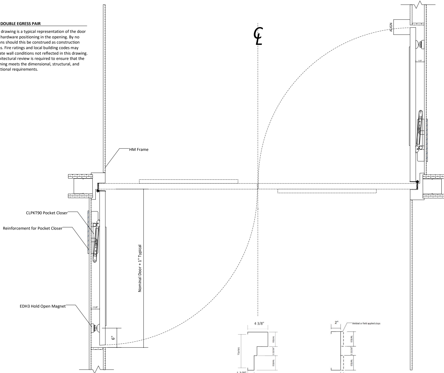
2 Jamb Detail Example (NTS)
