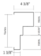
2 Jamb Detail Example (NTS)
